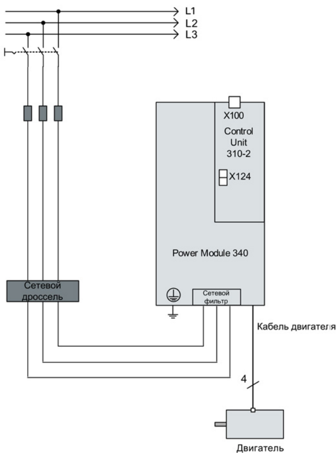
Изображение 3-32 Разводка компонентов (пример)
