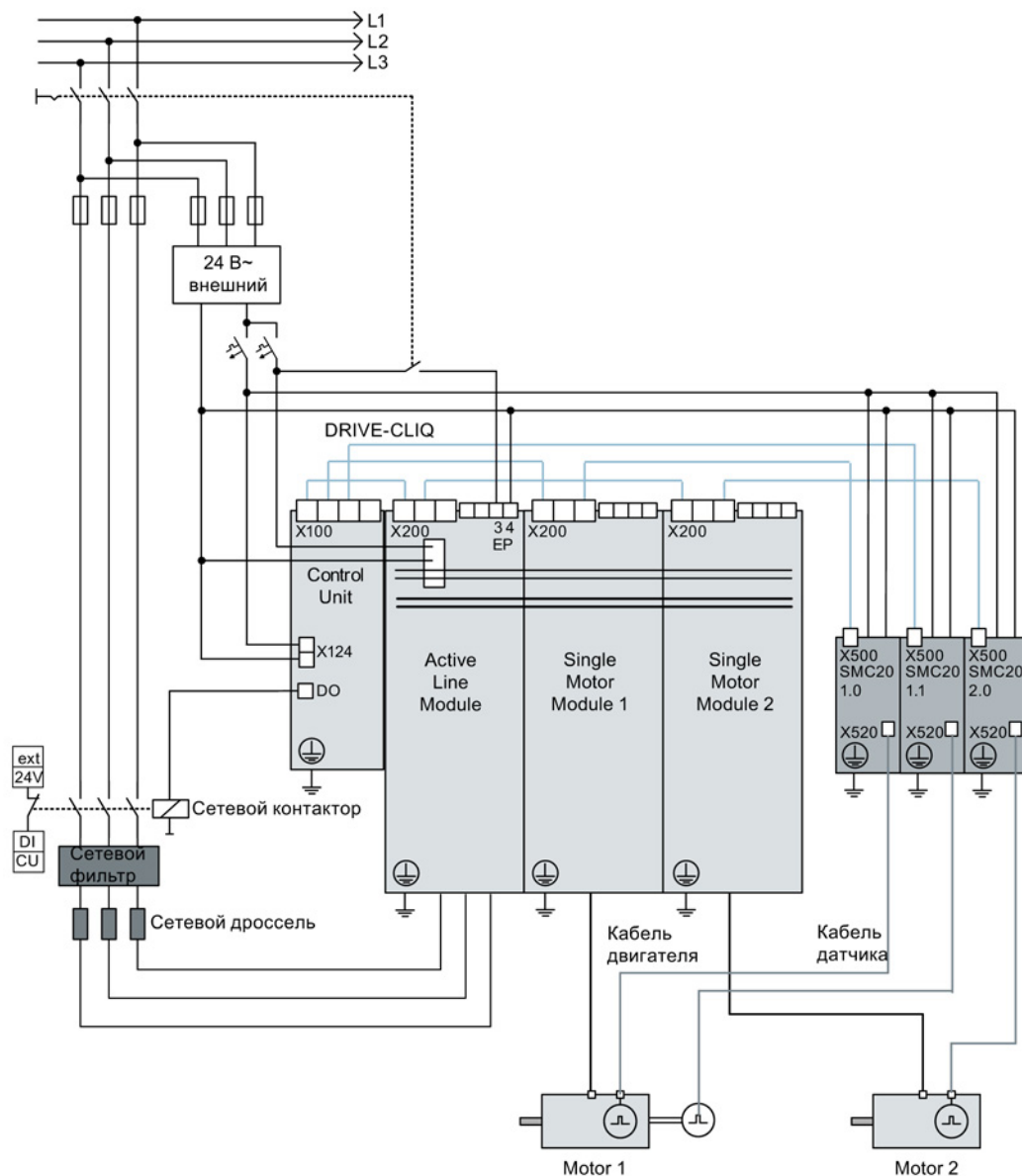
Изображение 3-25 Разводка компонентов (пример)
