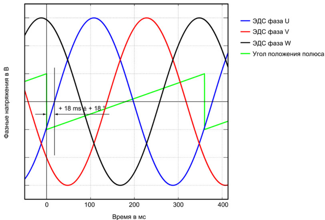
Изображение 3-67 Пример неправильно скомутированного привода
