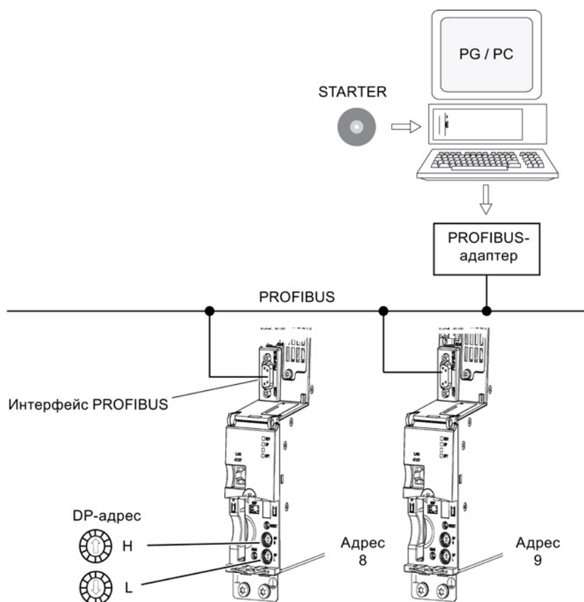
Изображение 3-13 Соединение программатора с целевым устройством через PROFIBUS
