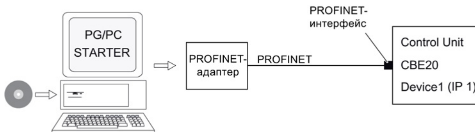
Изображение 3-19 Соединение программатора с целевым устройством через PROFINET (пример)
