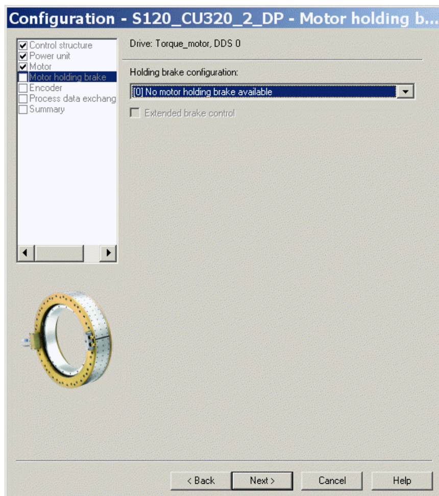
Изображение 3-77 Форма для конфигурации стояночного тормоза двигателя
