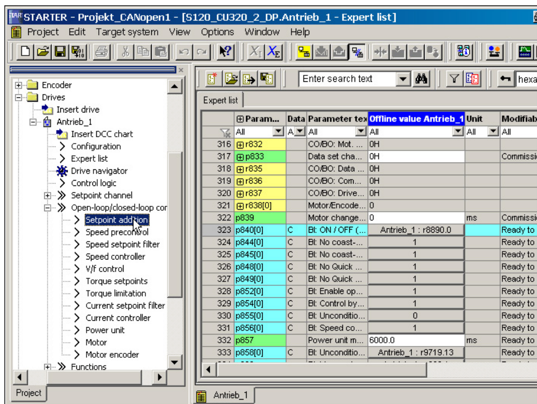
Изображение 3-6 Параметры в экспертном списке
