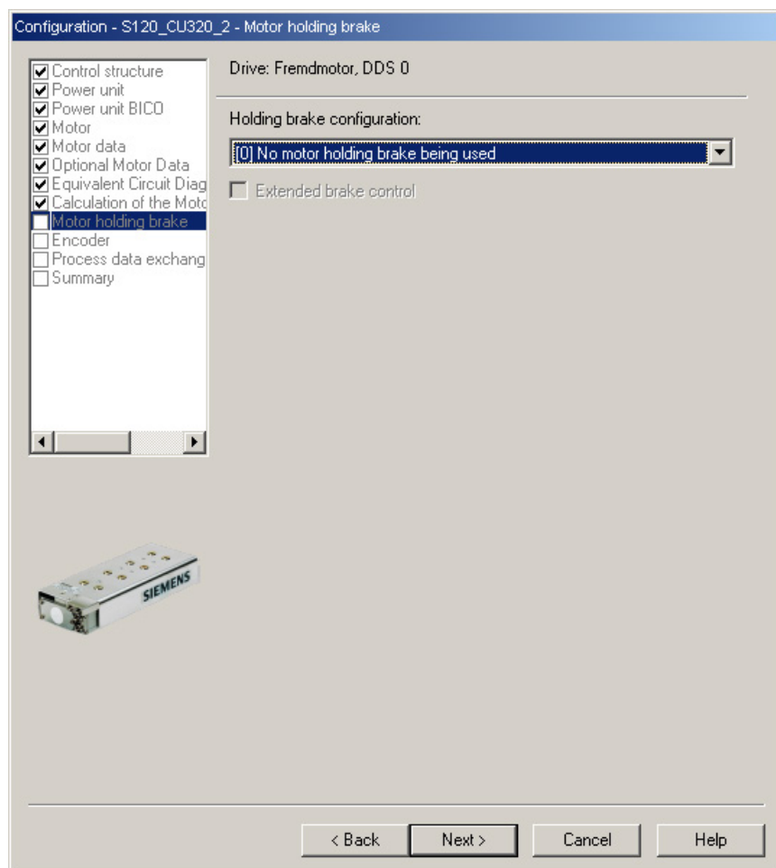
Изображение 3-48 Форма для конфигурации стояночного тормоза двигателя
