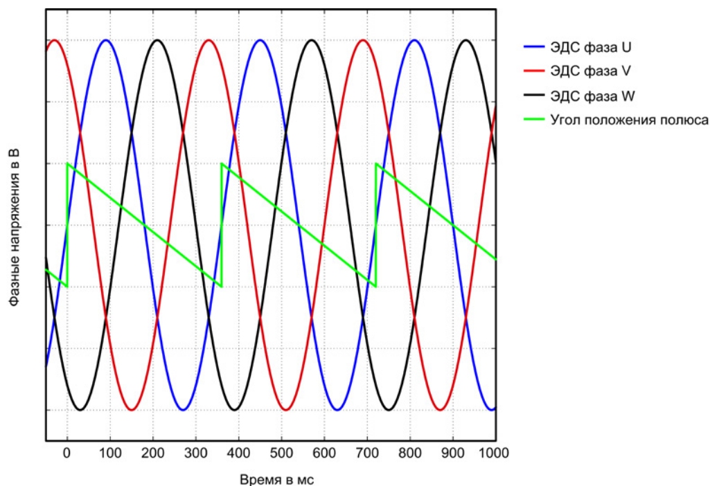
Изображение 3-65 ЭДС при отрицательном направлении движения
