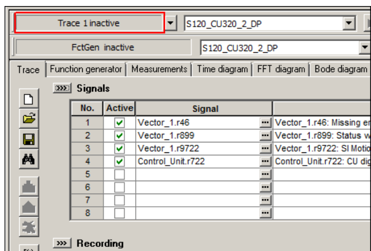
Изображение 4-7 Статус трассировки в STARTER
