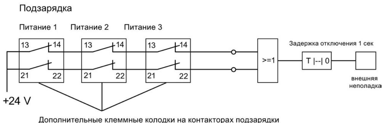
Изображение 3-36 Контроль контактора подзарядки
