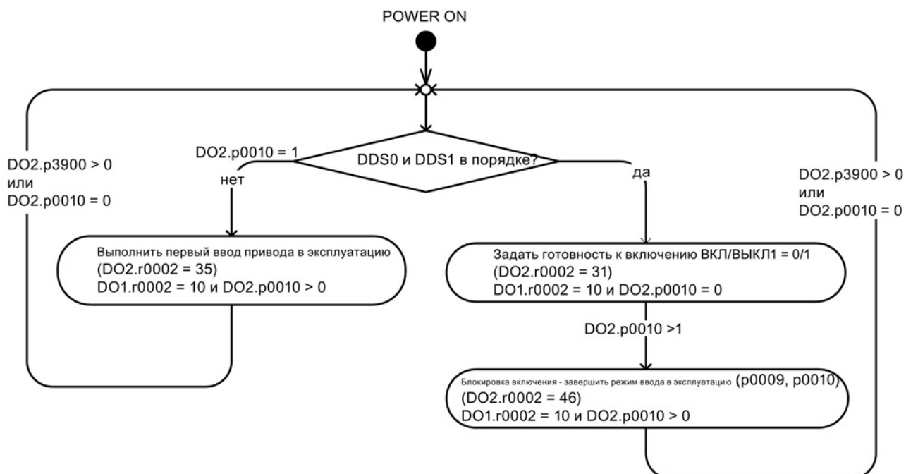
Изображение 4-13 Диагностика не введенных в эксплуатацию осей
