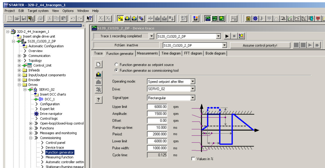
Изображение 4-3 Генератор функций
