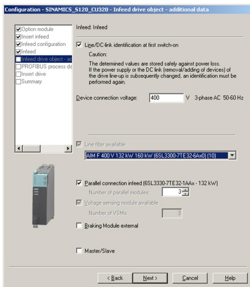
Изображение 3-34 Пример параллельного включения 3 активных модулей питания (формат «шасси»)
