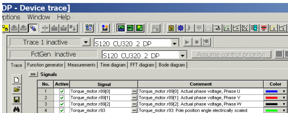
Изображение 3-91 Назначение каналов трассировки для проверки смещения угла коммутации
