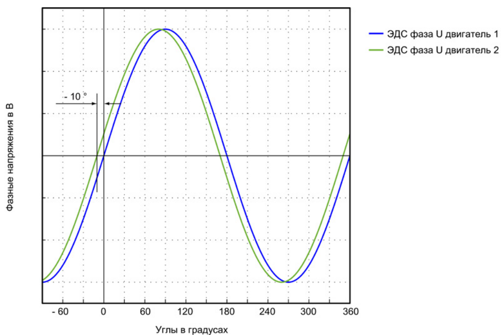
Изображение 3-87 Фаза U двигателя 1 может отставать от ЭДС фаза U двигателя 2 не более чем на 10^\circ
