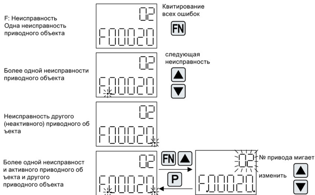
Изображение 3-103 Неполадки
