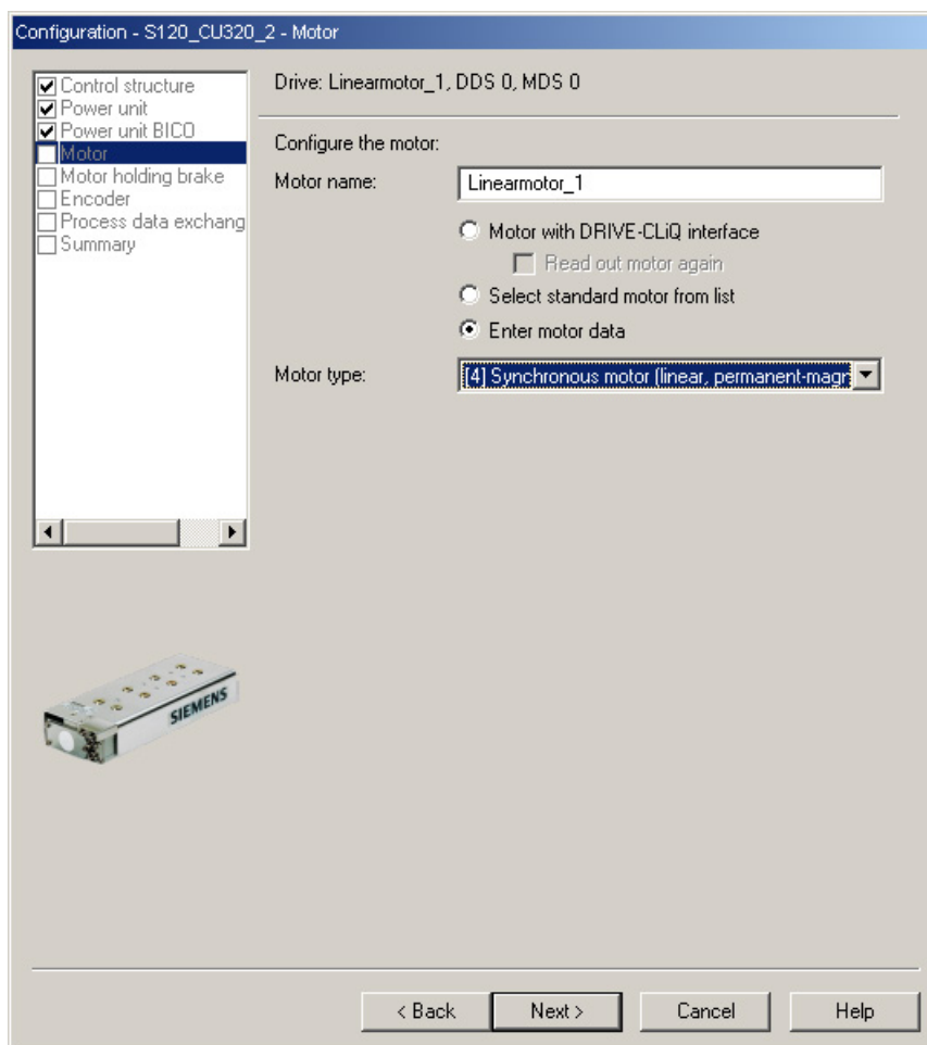
Изображение 3-43 Окно конфигурации двигателя – настройки двигателя стороннего производителя
