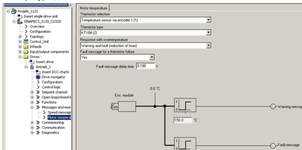
Изображение 3-97 Выбор датчика температуры для модулей SME20
